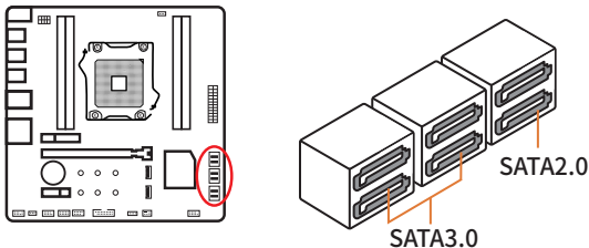
图2 -11 SATA接口
